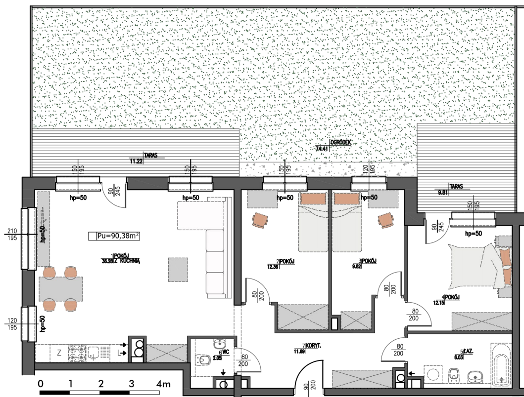
Rzut kondygnacji (parter):
